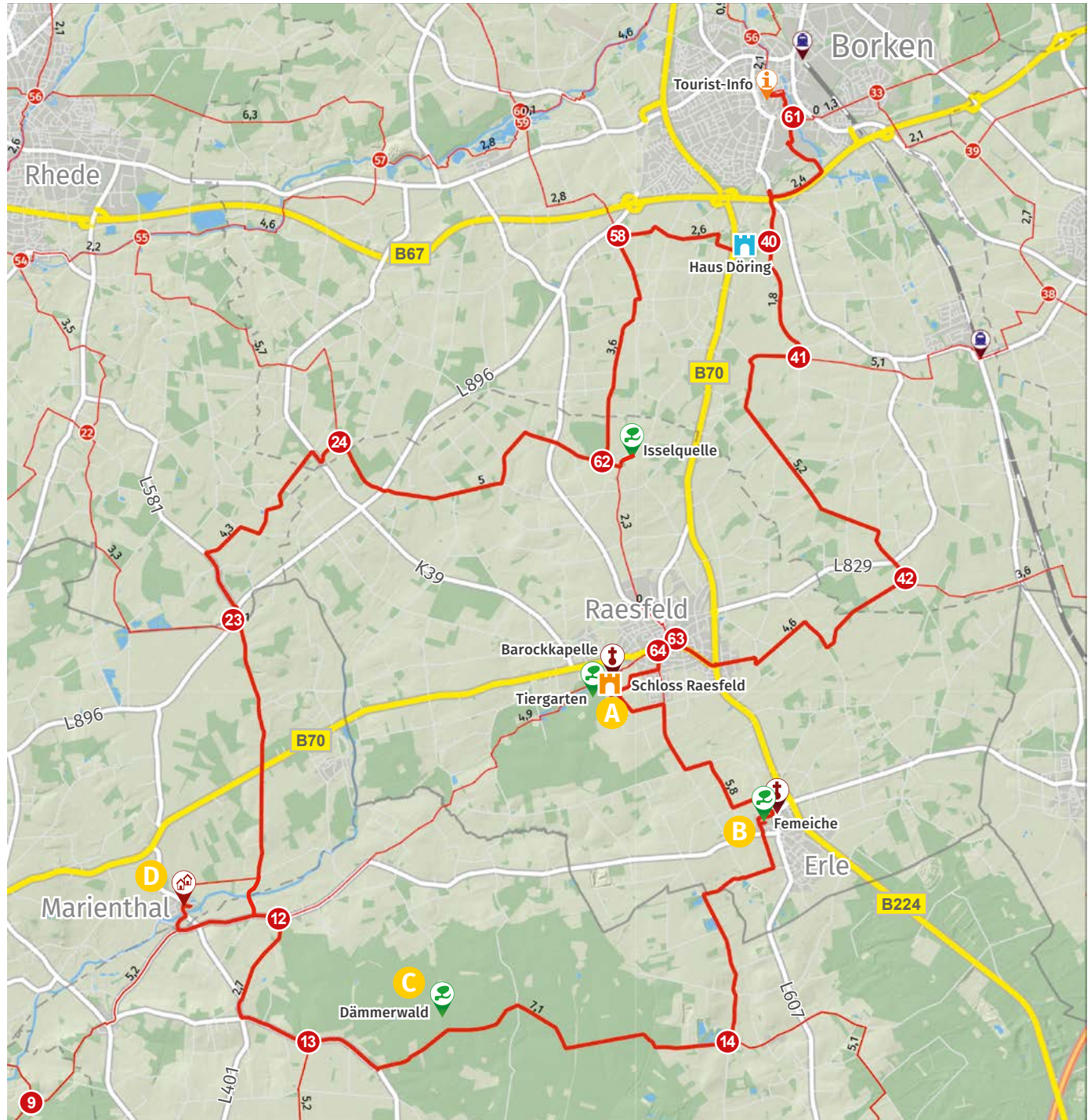
Auflistung Knotenpunkte: 61 40 41 42 63 64 (12) 64 14 13 12 (9) (12) 23 24 62 (63) 62 58 40 61
